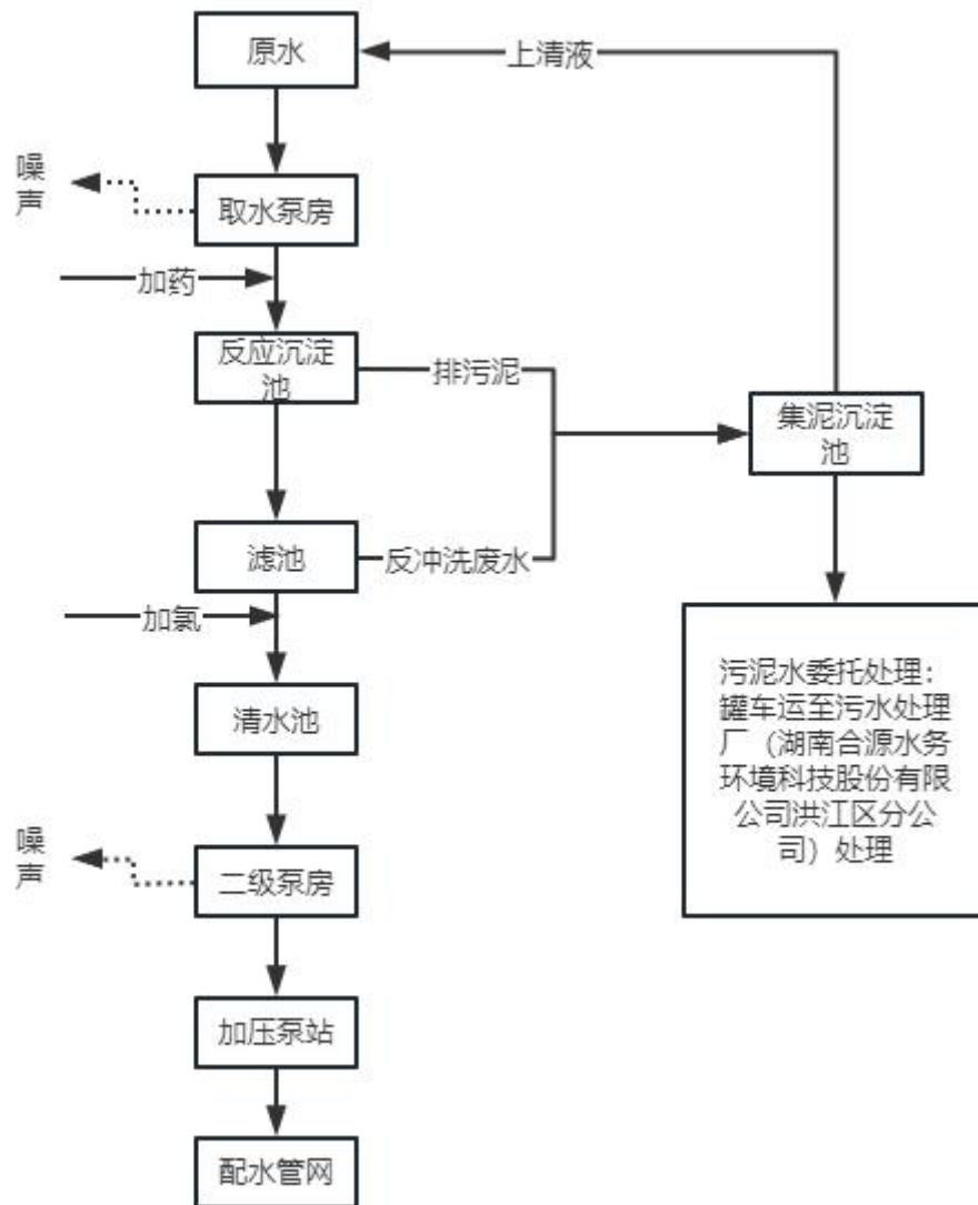
图2-4 改建后生产工艺流程及污染节点简图
