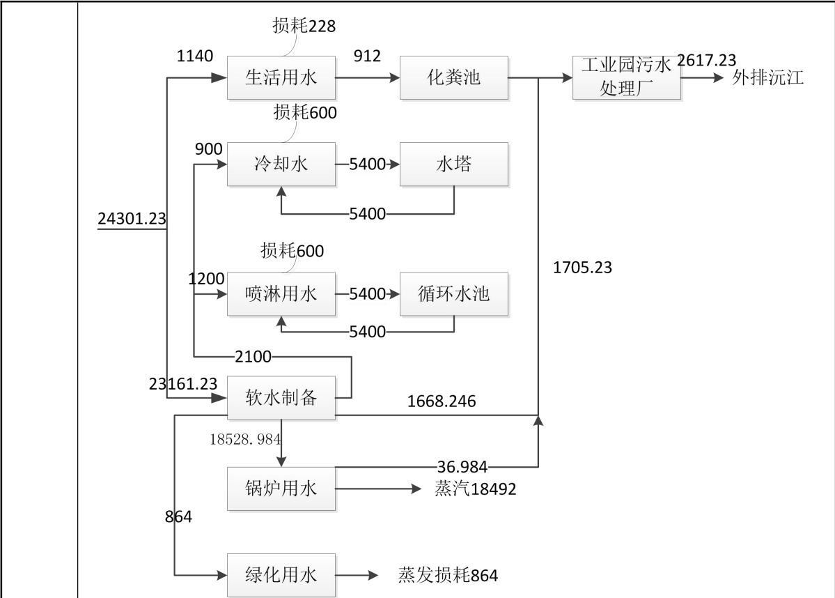
图 2-1 项目给排水平衡图（一期+二期） 单位：t/a
