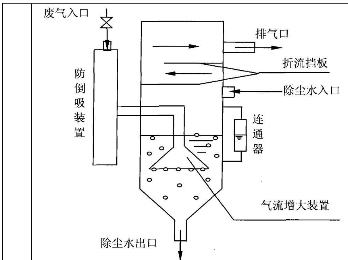
图 4-2 水喷淋式除尘器结构图
