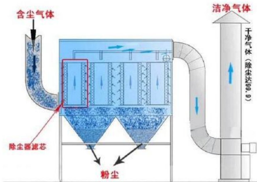
图 4-3 袋式除尘器结构图
